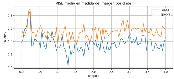
(b) Resultados de “margin” usando RISE.
