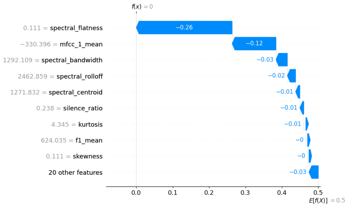
Figura 3.2: Explicación local con SHAP
